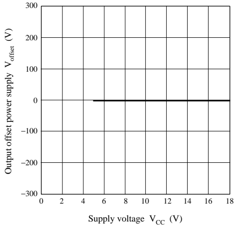
V_{OFFSET} — V_{CC}
